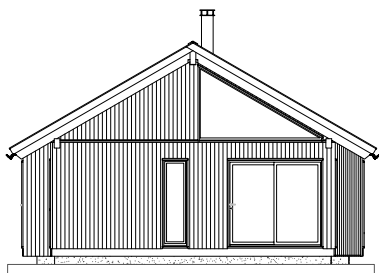
FASADE - ØST
