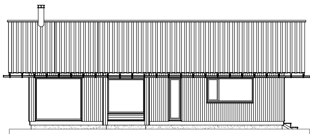
FASADE - SYD
