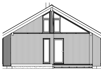
FASADE - VEST
