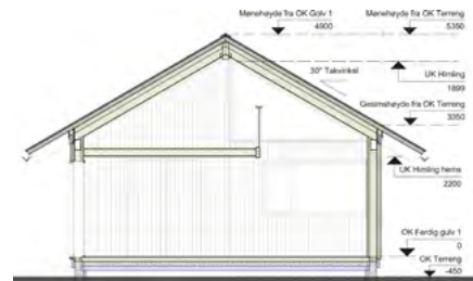
SNITT
