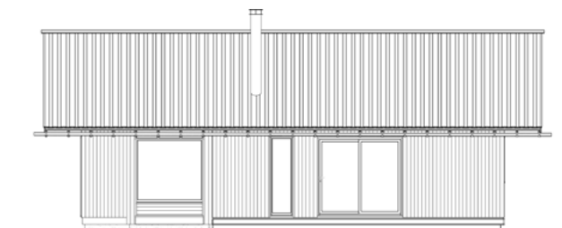
FASADE - NORDVEST
