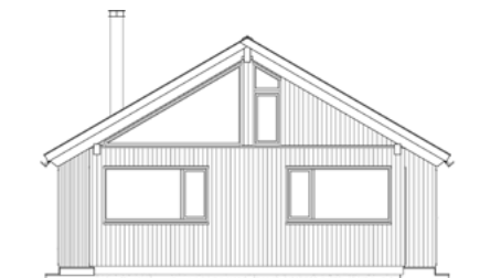
FASADE - SØRVEST
