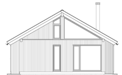
FASADE - NORDØST
