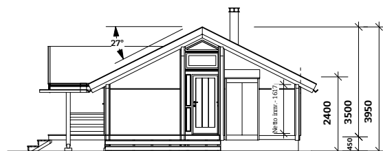
SNITT
